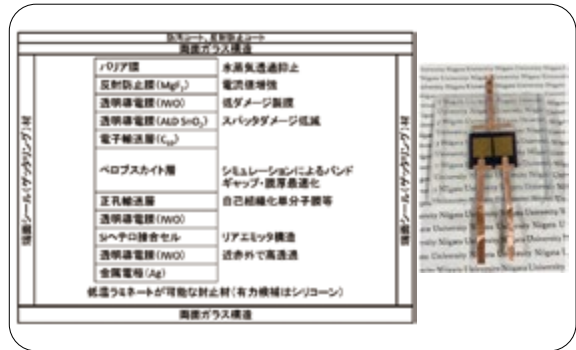
タンデム太陽電池の構造と課題
