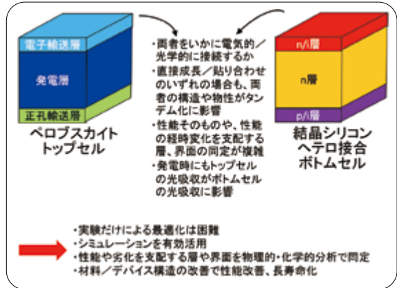
タンデム太陽電池の構造と課題
