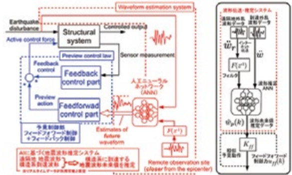
図1: 提案する制御系
