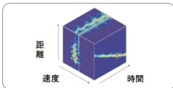
図2: ターゲットの距離・時間・速度特性
