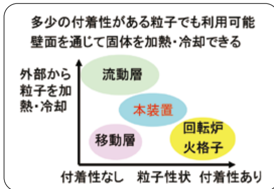
図2 本形式の気固接触装置の位置づけ
