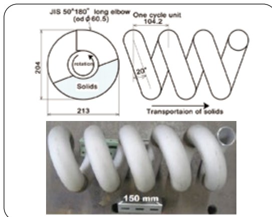
図1 らせん型気固接触装置の設計とその金属製試作品の例
