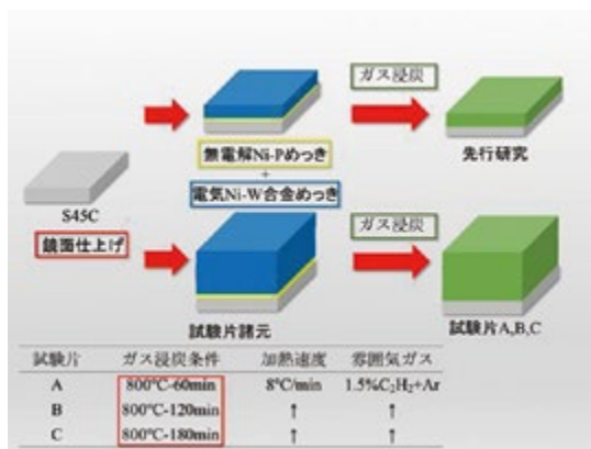
湿式めっき・ガス浸炭複合法によるWC-Ni硬質皮膜形成プロセス
