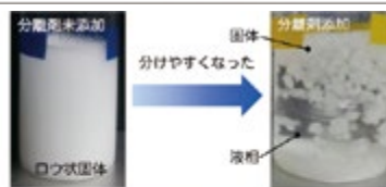
実験例：パルミチン酸メチル割合濃度と曇り点変化(0.5wt%添加)
