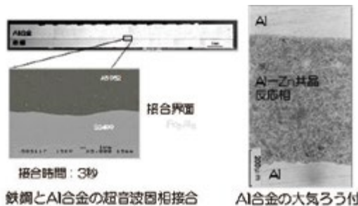
鉄鋼とAl合金の超音波固相接合 Al合金の大気ろう付 異種金属接合のマイクロ組織の例
