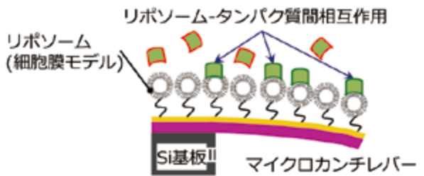
図2 タンパク質検知用バイオセンサへの応用
