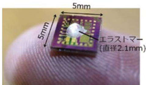
図1 試作した触覚センサチップ
