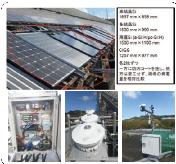
屋外曝露サイトの外観、発電量評価装置と気象測器
