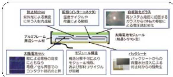
従来型太陽電池モジュールの劣化機構と問題点
