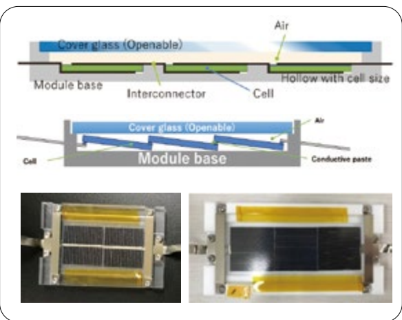
本研究で提案するモジュール構造と外観
