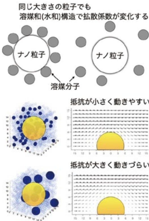
2成分溶媒中における粒子周りの溶媒の速度場。速度場は溶媒和構造によって決まり、粒子の動きやすさに影響する。
