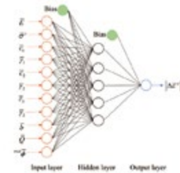
ニューラルネットワークの構成 [図2]
