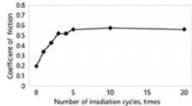
図2 レーザ照射による高摩擦表面と摩擦係数
