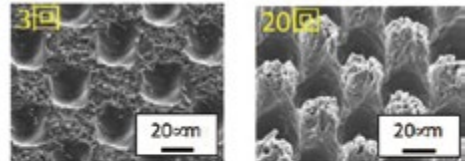
図1 高摩擦係数表面による小型化の例
